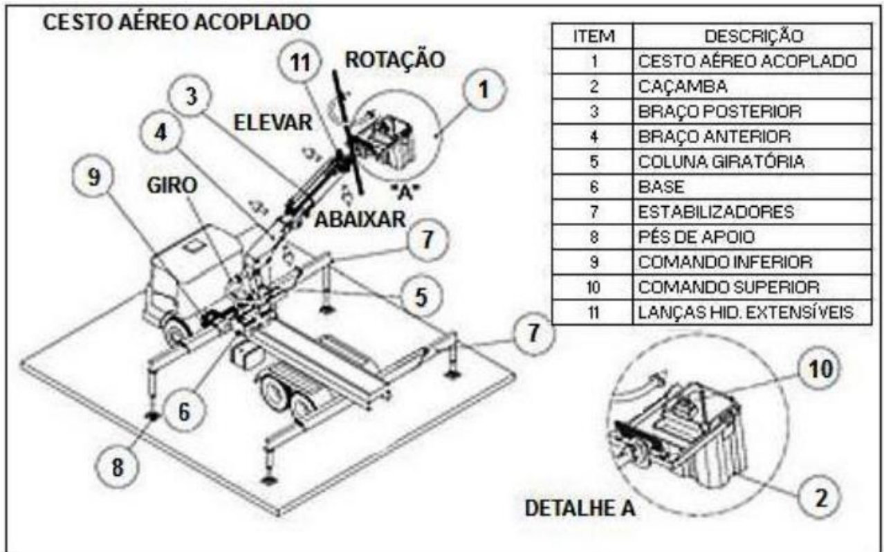
Figura 1 - Exemplo de Arranjo de um Cesto Aéreo Acoplado
