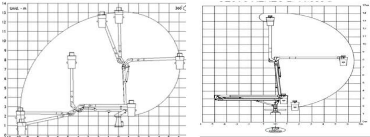
Figuras 2 e 3 – Diagrama Operacional
